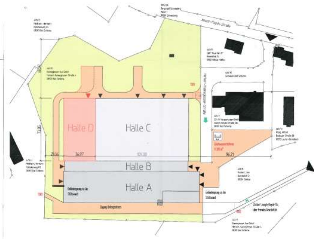
Grundriss Hallenkomplex, Auszug Bauvoranfrage
