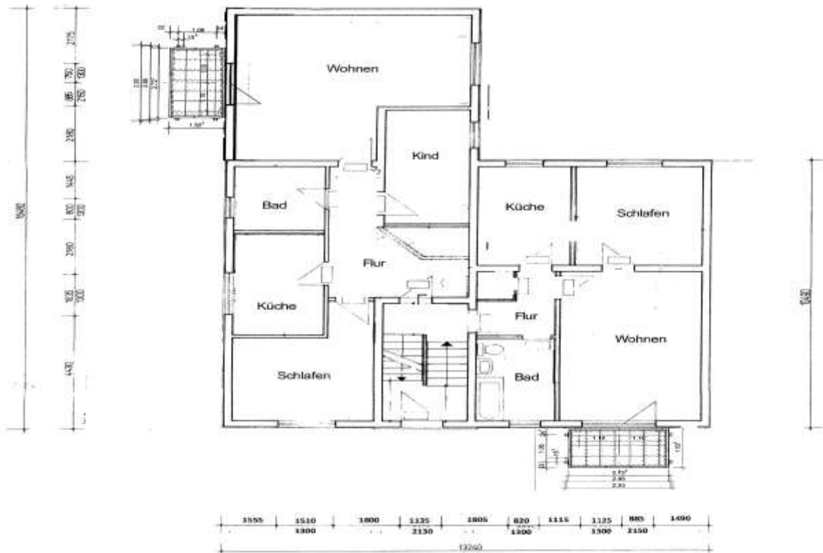
Auszug Grundriss Erdgeschoss zum Bauantrag, Friedrich-Gottlob-Straße 1
