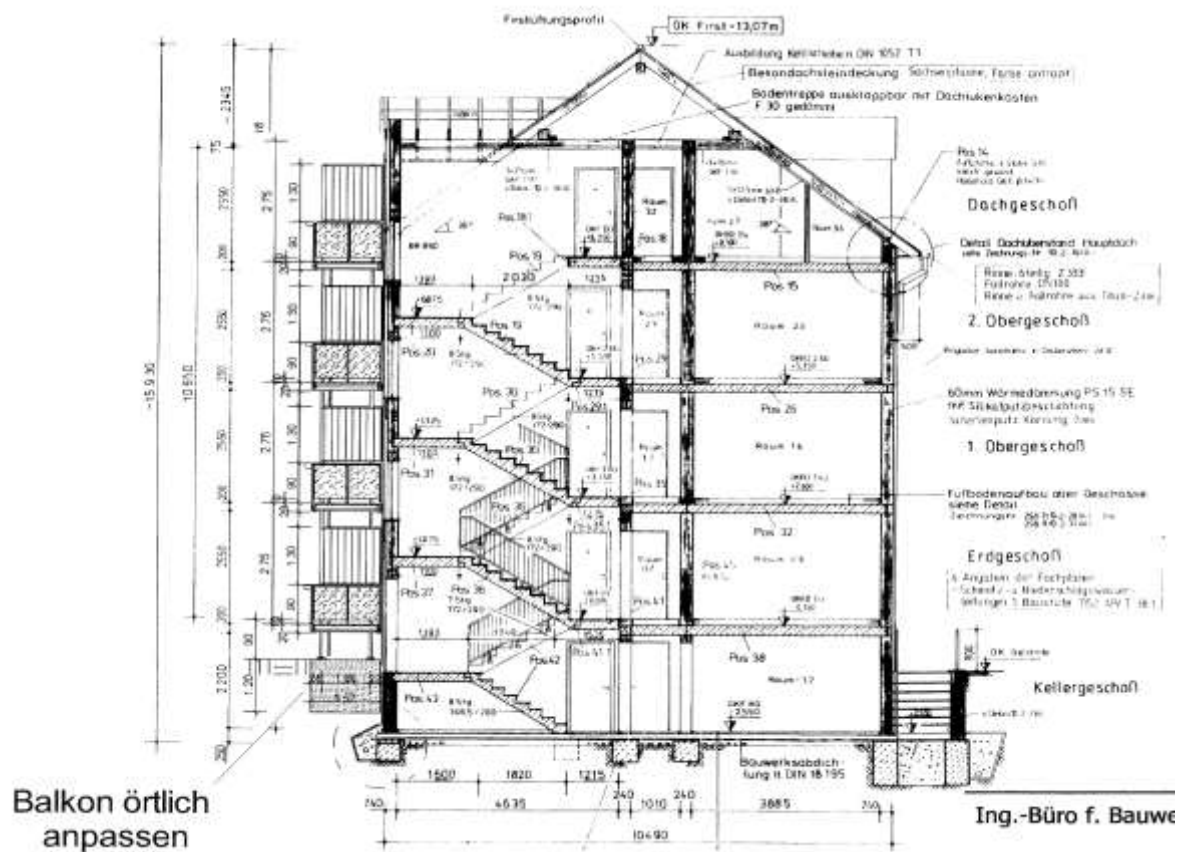
Auszug Schnitt zum Bauantrag, Friedrich-Gottlob-Keller-Straße 7
