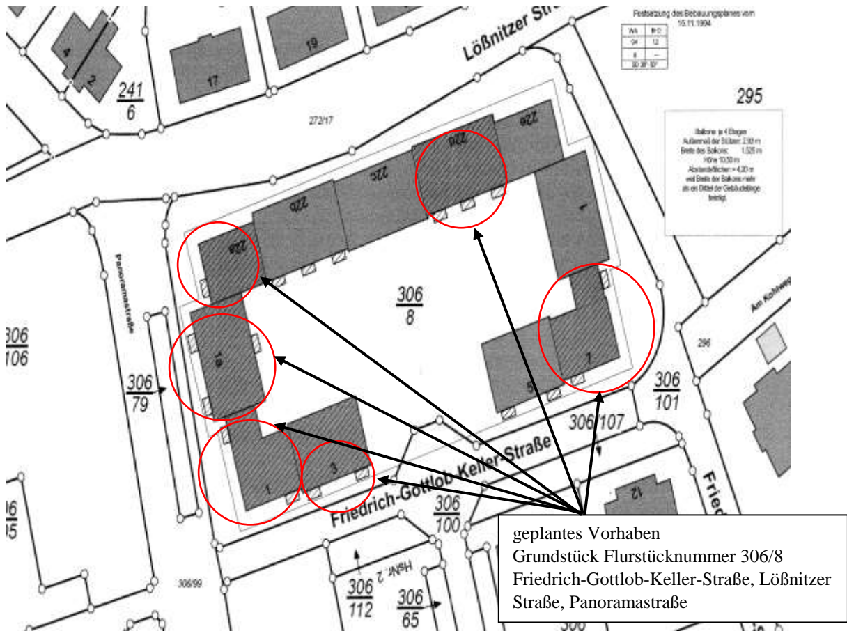
Auszug Lageplan für Balkone zum Bauantrag
