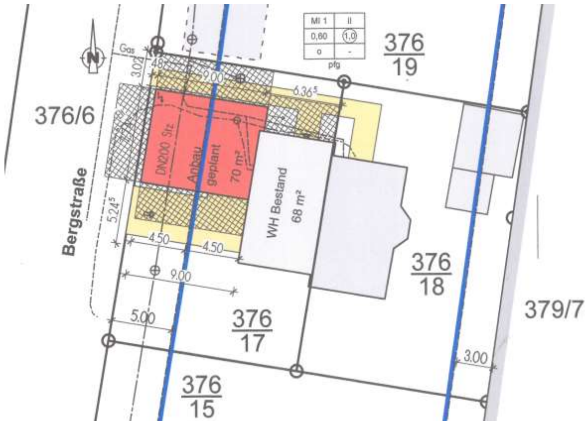
Auszug Lageplan zum Bauantrag – 1. Tektur
