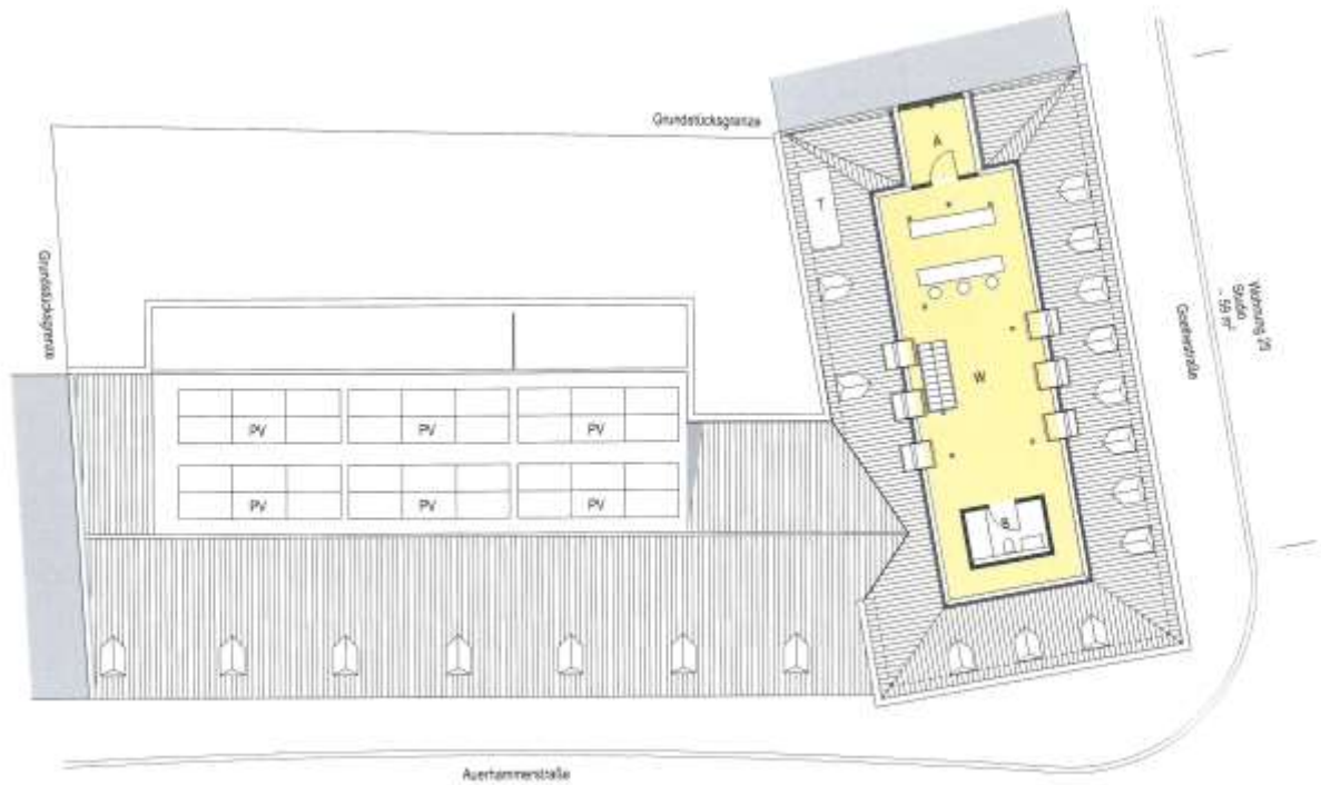
Auszug Grundriss 4. Obergeschoss zur Bauvoranfrage
