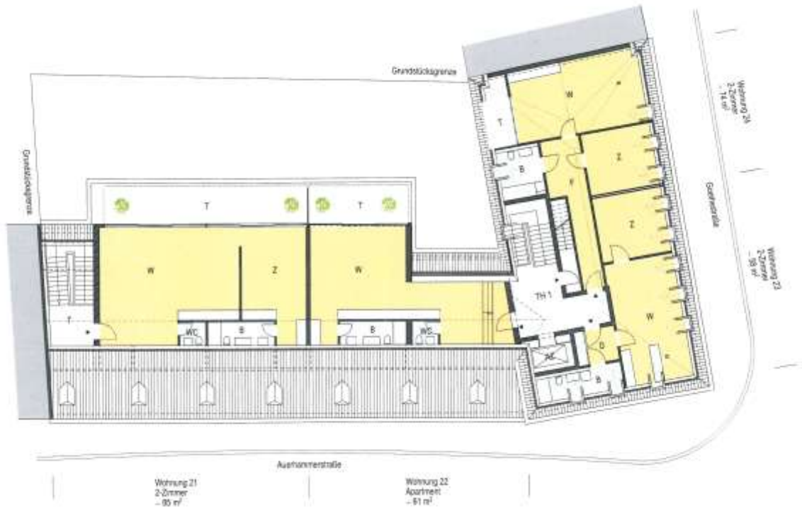
Auszug Grundriss 4. Obergeschoss zur Bauvoranfrage
