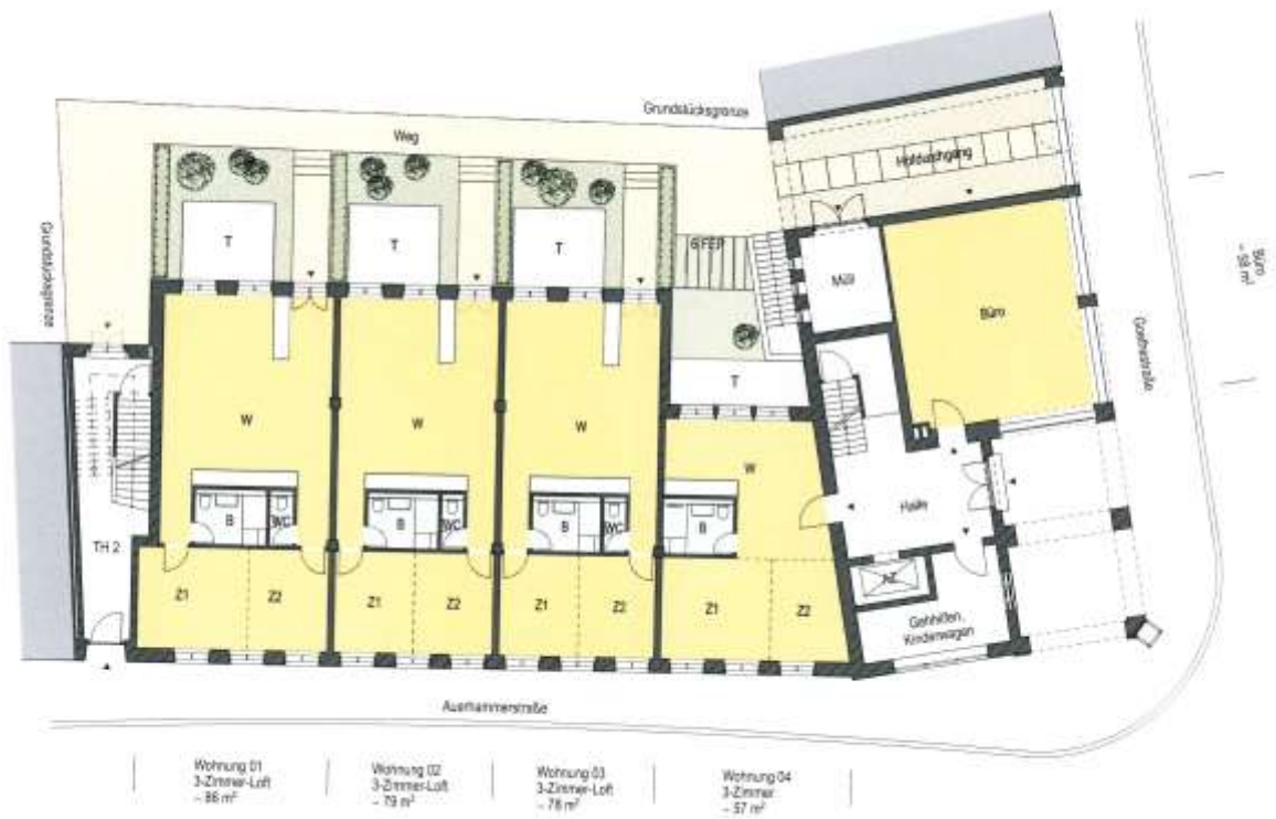
Auszug Grundriss Erdgeschoss zur Bauvoranfrage
