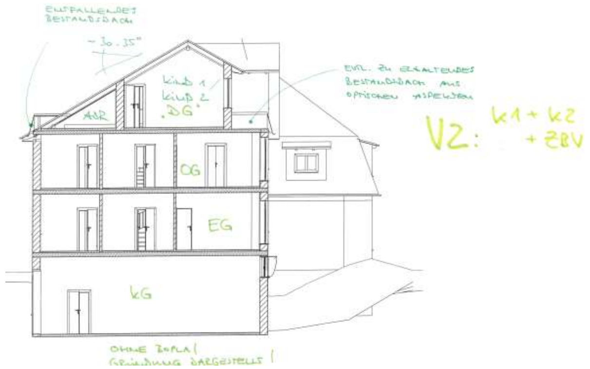
Auszug Schnitt zur Bauvoranfrage
