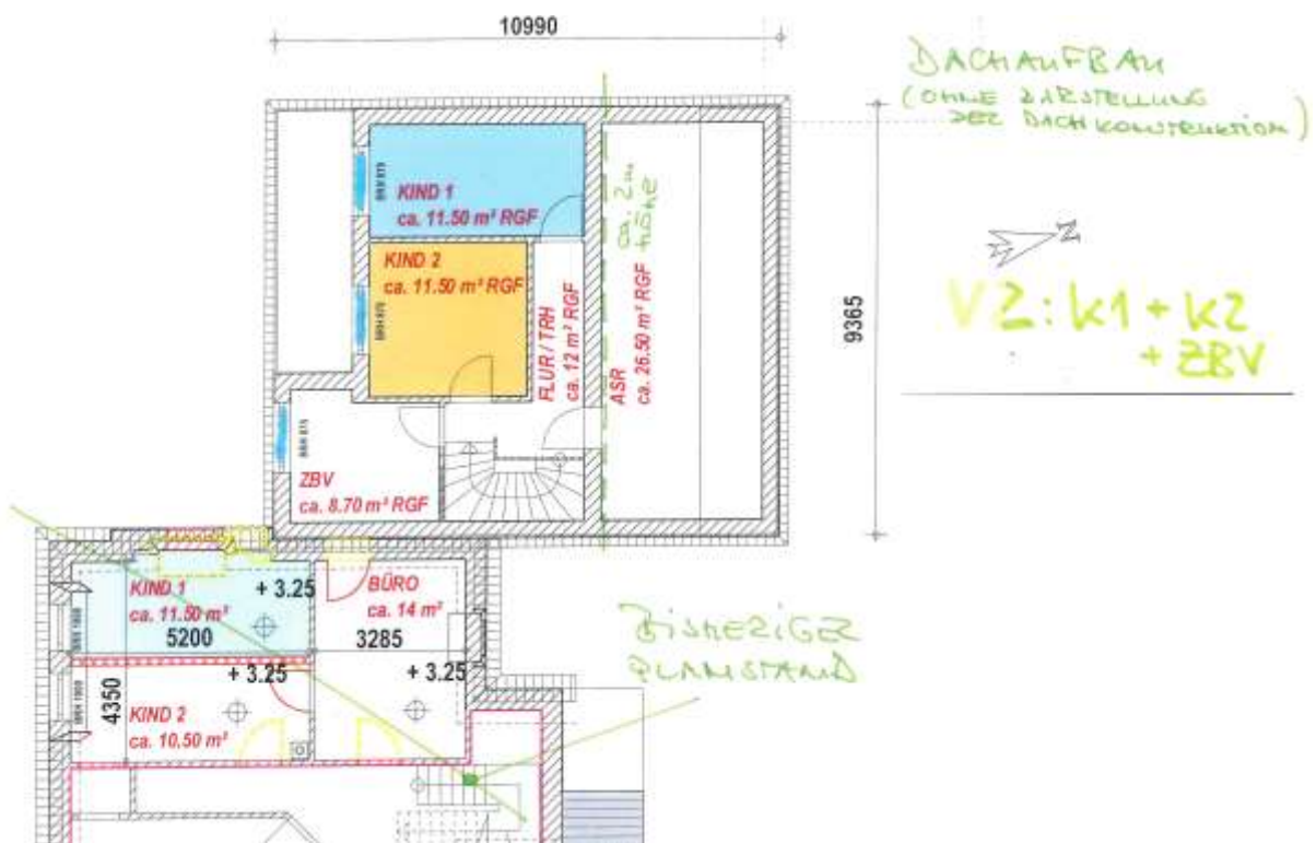
Auszug Grundriss Dachgeschoss zur Bauvoranfrage
