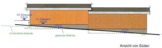
Auszug Ansichten Carportanlage zum Bauantrag (oben links – Ansicht von Norden, oben rechts – Ansicht von Osten, unten links – Ansicht von Süden, unten rechts – Ansicht von Westen)
