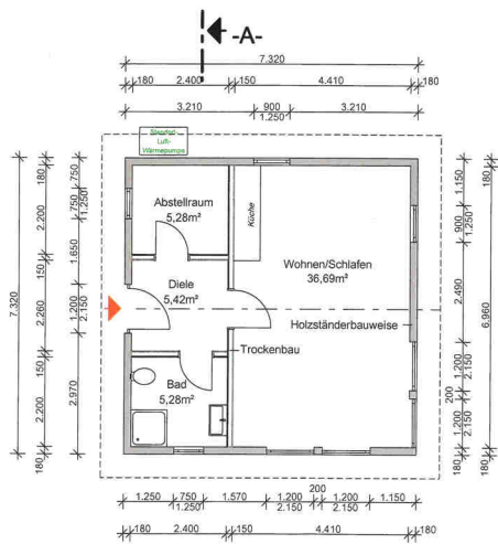
Auszug Grundriss Erdgeschoss (links) und Schnitt (rechts) Wohngebäude
