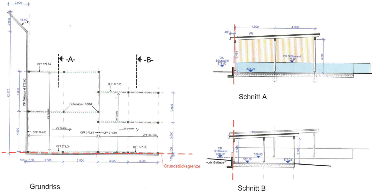
Auszug Grundriss (links) und Schnitt (rechts) Carportanlage
