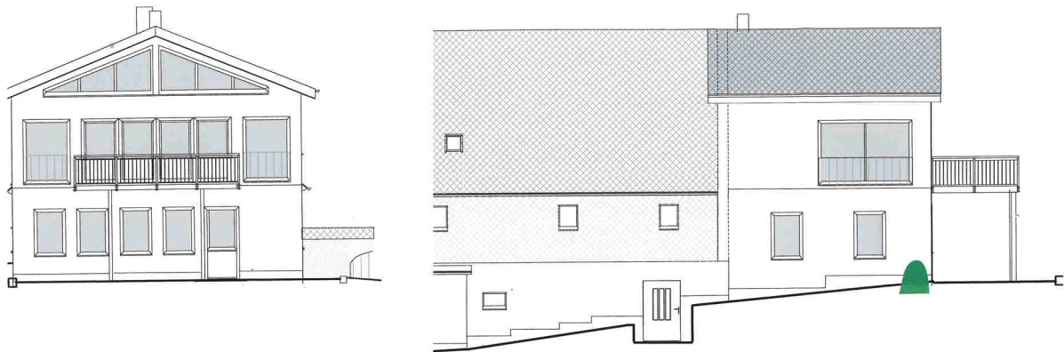
Auszug Ansichten Wohngebäude zum Bauantrag (links – Ansicht von Süd, rechts – Ansicht von West)
