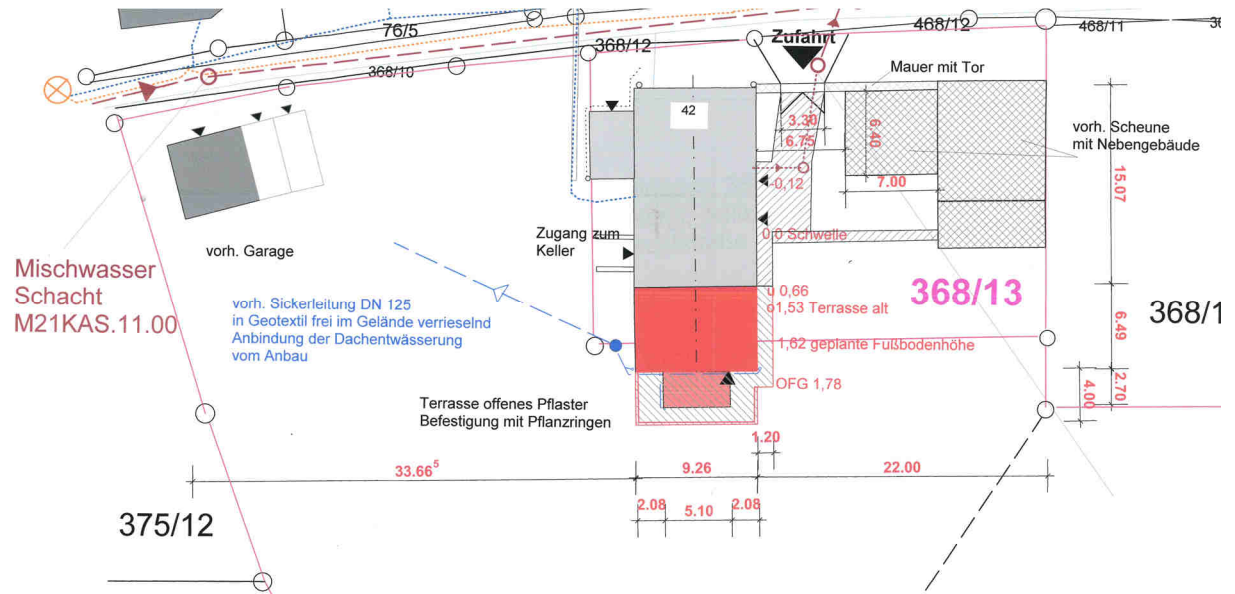
Auszug Lageplan zum Bauantrag
