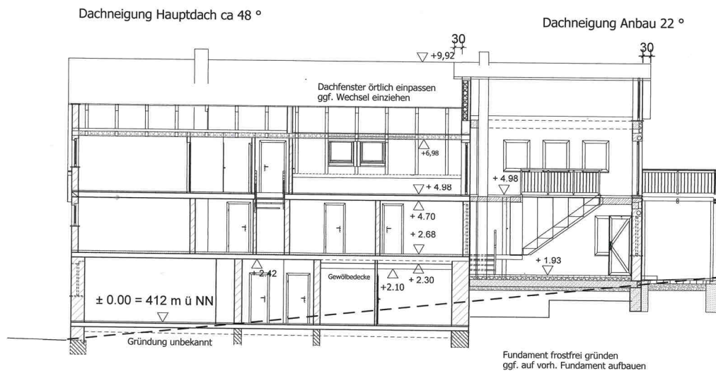
Auszug Längsschnitt zum Bauantrag
