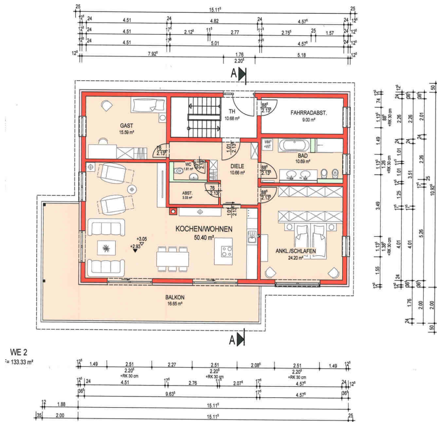
Auszug Grundriss Obergeschoss zum Bauantrag
