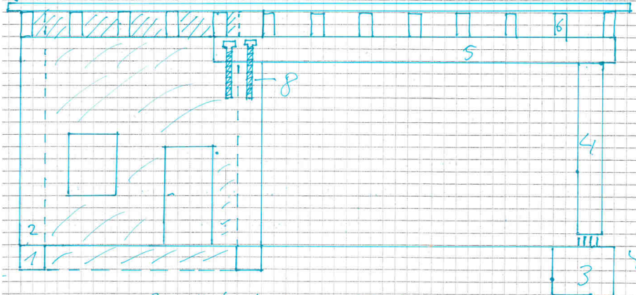
Auszug Schnitt zum Bauantrag
