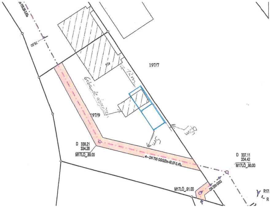
Auszug Lageplan zum Bauantrag
