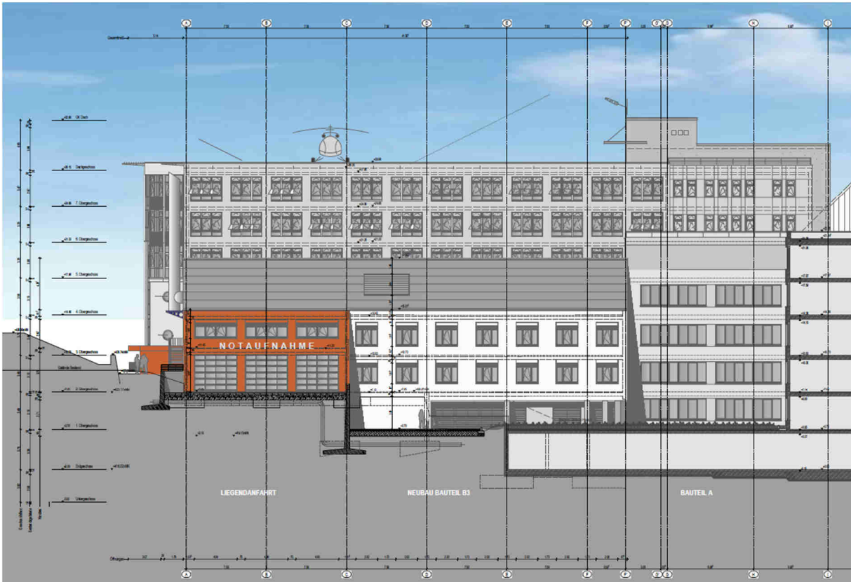
Auszug Ansicht von Nord-West zum Bauantrag
