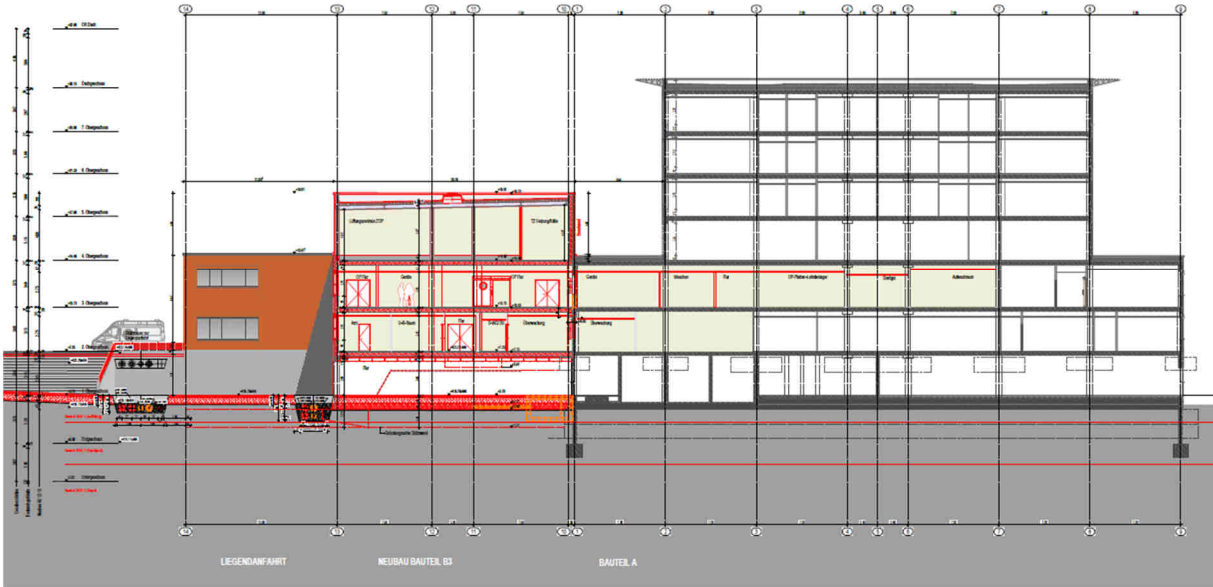
Auszug Schnitt zum Bauantrag
